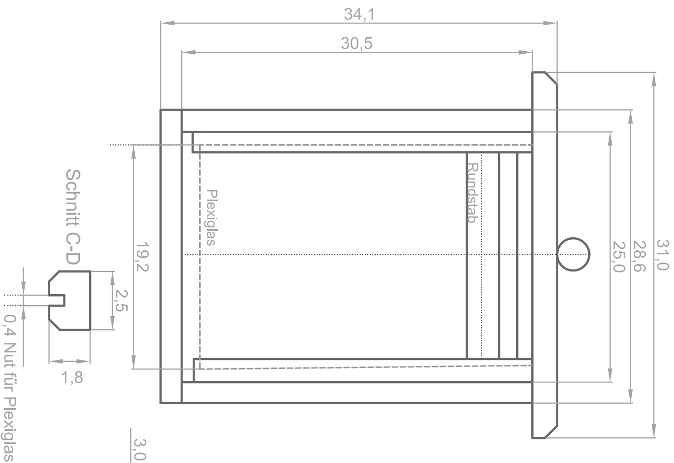
Vorderansicht
